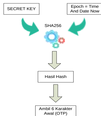
Gambar 3. Proses Pengambilan 6 Karakter Awal OTP
