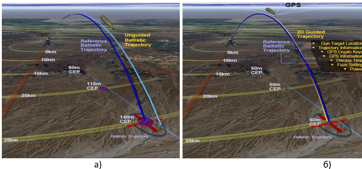
Рис.8. Траєкторії руху ОФ снаряду:
