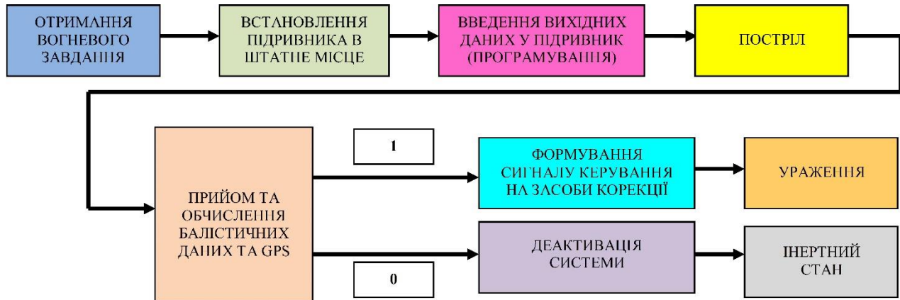
Схема 1. Послідовність роботи багатофункціонального підривника з GPS-корекцією
