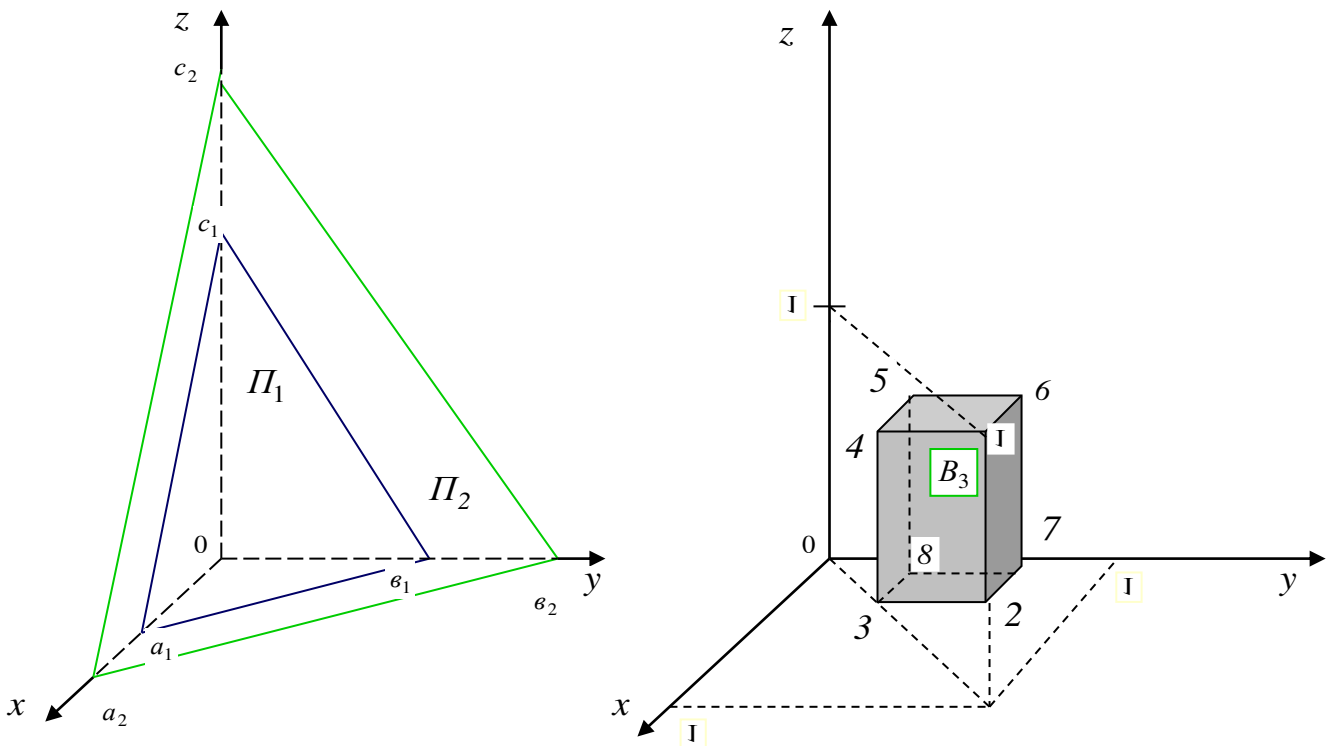
Рис. Ілюстрація вирішення задачі розподілу допусків у термінах аналітичної геометрії у просторі
