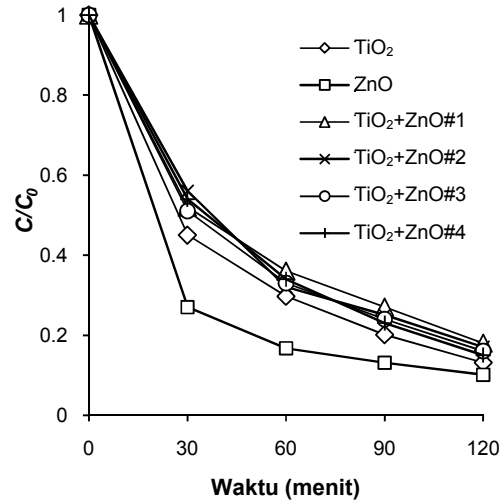
Gambar 8. Dekolorisasi fotokatalitik AR4 dengan kombinasi katalis \text{TiO}_2 dan \text{ZnO} ([AR4]: 10 mg/L, pH 11, [total katalis]:0,5 g/L)
