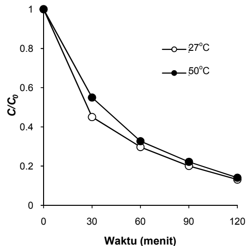
Gambar 10. Dekolorisasi fotokatalitik AR4 dengan pengaruh temperatur ([AR4]: 10 mg/L, pH 11, [TiO 2 ]: 0,5 g/L)
