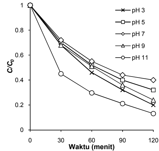
Gambar 4. Dekolourisasi fotokatalitik AR4 dengan katalis TiO 2 dengan variasi pH ([AR4]: 10 mg/L, [TiO 2 ]: 0,5 g/L)
