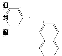
Gambar 1. Struktur molekul Acid Red 4
