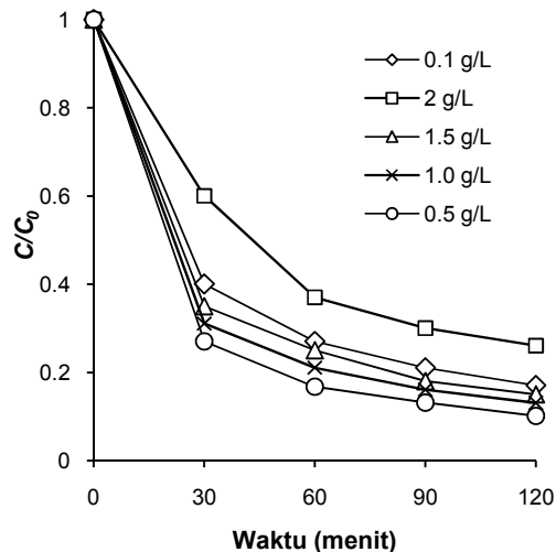
Gambar 7. Dekolorisasi fotokatalitik AR4 dengan variasi dosis katalis ZnO ([AR4]: 10 mg/L, pH 11).
