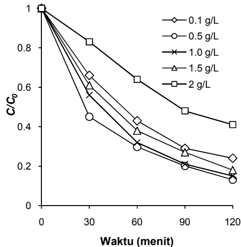
Gambar 6. Dekolorisasi fotokatalitik AR4 dengan variasi dosis katalis TiO 2 ([AR4]: 10 mg/L, pH 11)
