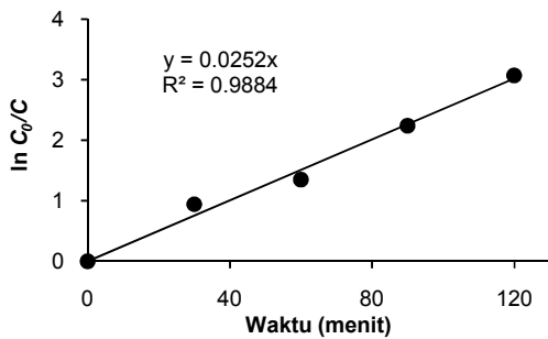
Gambar 3. Laju dekolourisasi mengikuti persamaan kinetika pseudo orde pertama ([AR4]: 10 mg/L, [TiO 2 ]: 0,5 g/L).
