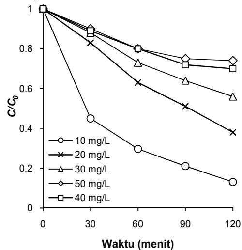
Gambar 5. Dekolorisasi fotokatalitik AR4 dengan katalis TiO 2 dengan variasi konsentrasi awal warna ([TiO 2 ]: 0.5 g/L, pH 11)
