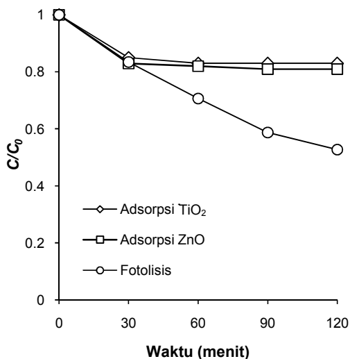
Gambar 9. Dekolorisasi AR4 dengan pengaruh adsorpsi dan fotolisis ([AR4]: 10 mg/L, pH: 11, [TiO 2 ]: 0,5 g/L)
