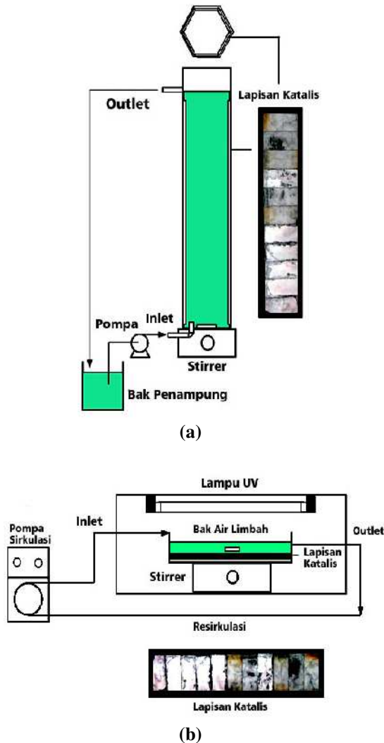
Gambar 2. Diagram skematik reaktor: (a) reaktor vertikal; (b) reaktor horisontal
