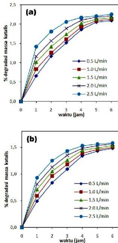
Gambar 5. Degradasi massa katalis pada berbagai variasi laju alir fluida: (a) katalis nanofiber; (b) katalis komposit
