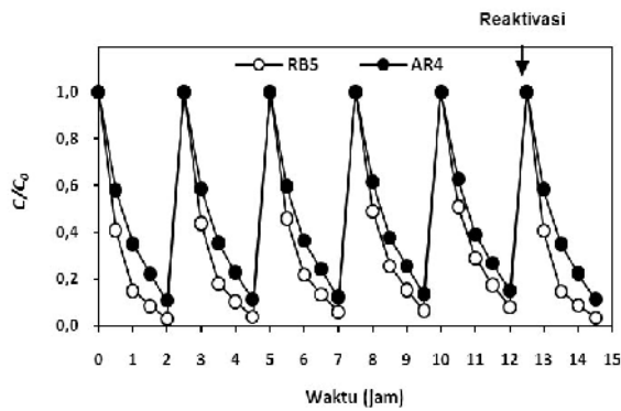
Gambar 9. Penggunaan ulang katalis terhadap air limbah simulasi (a) RB5; (b) AR4 (kons. zw.: 30 mg/L, kons. katalis: 2,0 g/L, pH 11)
