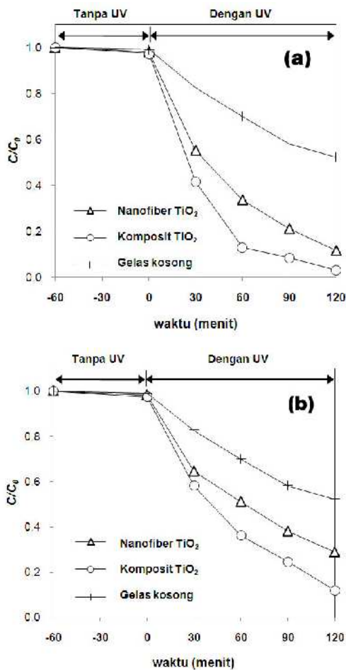
Gambar 7. Dekolorisasi warna oleh adsorpsi dan proses fotokatalitik oleh berbagai variasi fotokatalis terhadap air limbah simulasi: (a) RB5; (b) AR4 (kons. zw.: 10 mg/L, pH 11, kons. katalis: 2 g/L)
