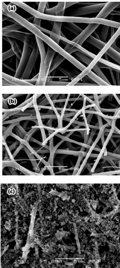
Gambar 3. Citra SEM (pembesaran 5000x): (a) nanofiber TiO 2 sebelum kalsinasi; (b) nanofiber TiO 2 setelah kalsinasi; (c) komposit nanofiber TiO 2 setelah kalsinasi
