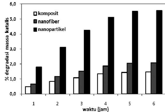
Gambar 4. Degradasi massa tiga jenis katalis oleh pengaruh aliran fluida (fluida: air suling, laju alir: 0,5 L/menit)
