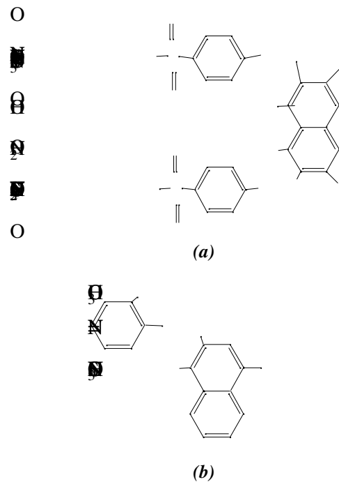
Gambar 1. Struktur molekul zat warna: (a) Reactive Black 5; (b) Acid Red 4
