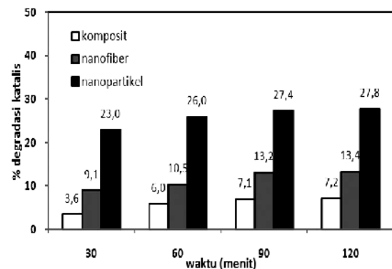
Gambar 6. Degradasi massa tiga jenis katalis oleh pengaruh sonikasi (fluida: air suling, frekuensi sonikator: 40 kHz, volume sonikator: 4 L)
