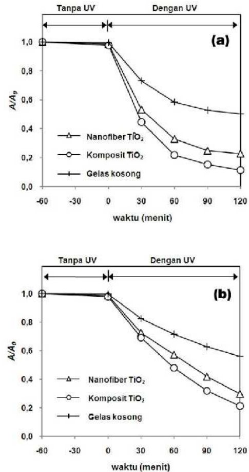
Gambar 8. Dekolorisasi warna oleh adsorpsi dan proses fotokatalitik oleh berbagai variasi fotokatalis terhadap efluen IPAL tekstil: (a) IPAL A; (b) IPAL B (kons. katalis: 2,0 g/L)
