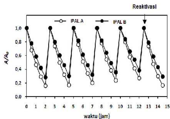
Gambar 10. Penggunaan ulang terhadap efluen IPAL tekstil: (a) IPAL A; (b) IPAL B (kons. katalis: 2,0 g/L).
