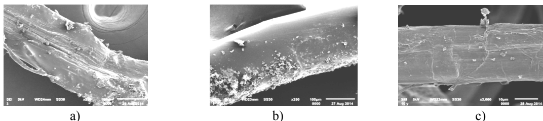
Gambar 8. Hasil uji SEM komposit serat alam + epoksi penampang membujur: a) serat rami, b) serat kelapa, c) serat abaka
