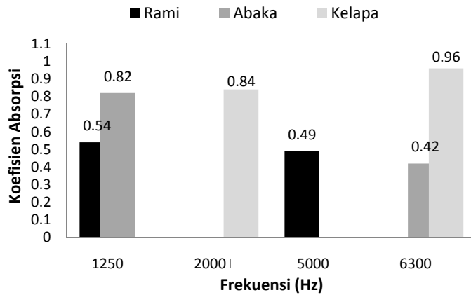
Gambar 5. Kondisi optimum koefisien absorpsi komposit serat alam pada frekuensi standar (1000Hz-4000Hz) dan frekuensi tinggi (5000 Hz-6300 Hz)
