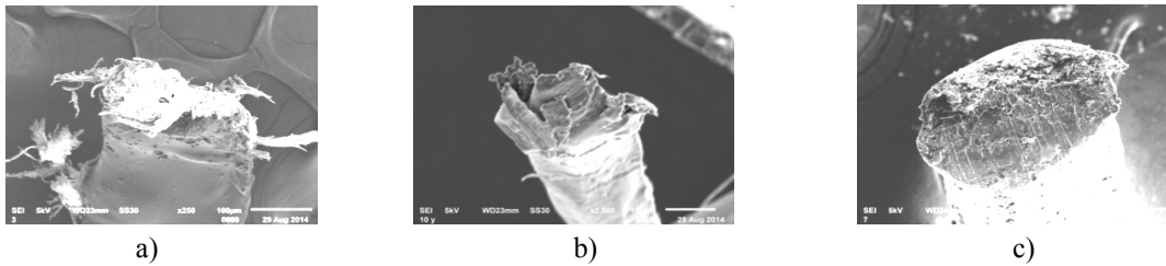
Gambar 9. Hasil uji SEM komposit serat alam + epoksi penampang melintang: a) serat rami, b) serat kelapa, c) serat abaka
