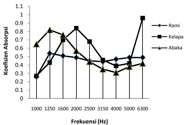
Gambar 6. Koefisien absorpsi suara ( \alpha ) Komposit Serat Rami, Kelapa Dan Abaka
