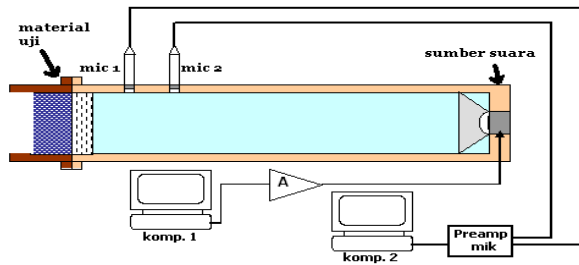
Gambar 1. Skema tabung impedansi
