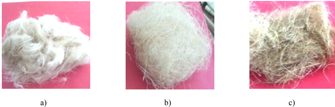
Gambar 2. Serat alam setelah proses degumming : a) serat rami, b) serat kelapa, c) serat abaka
