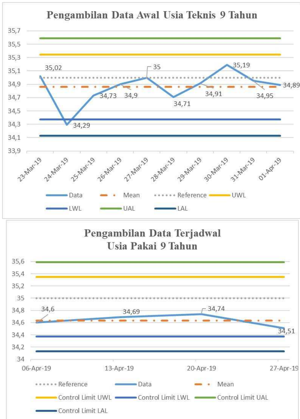
Gambar 5 Hasil grafik baby incubator B
