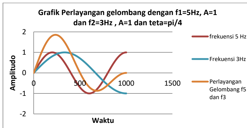
Gambar 7. Grafik Perlayangan gelombang dengan f_1 = 5 Hz dan f_2 = 3 Hz, A_1 = A_2 = 1 dan beda fase = \pi/4 (menggunakan Excel)
