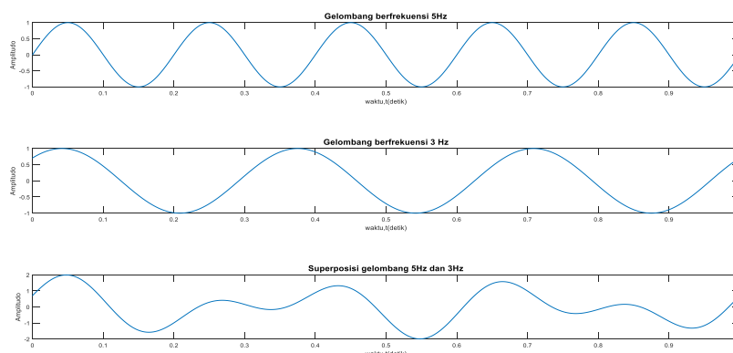
Gambar 8. Grafik Perlayangan gelombang dengan f_1 = 5 Hz dan f_2 = 3 Hz, A_1 = A_2 = 1 dan beda fase = \pi/4 (menggunakan Matlab)
