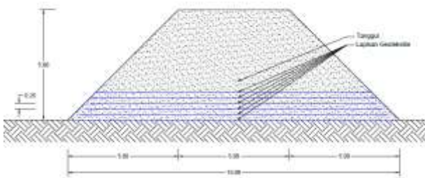
Gambar 5. Pemasangan geotekstil.
