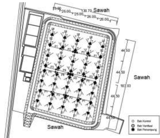
Gambar 15. Perencanaan jaringan pipa air lindi.
