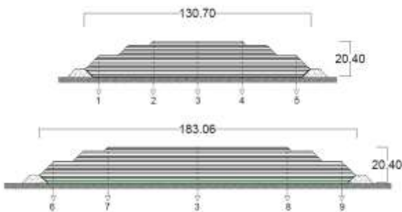
Gambar 9. Potongan melintang dan memanjang titik uji perhitungan pemampatan.
