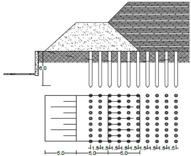
Gambar 14. Perkuatan cerucuk untuk timbunan sampah menghadap Kolan IPAL.
