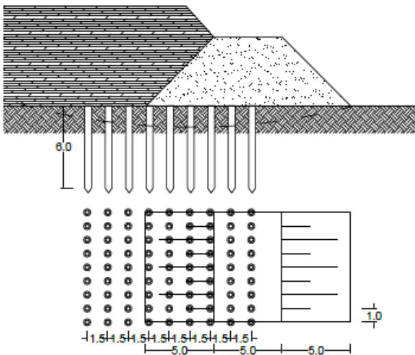
Gambar 13. Perkuatan cerucuk untuk timbunan sampah menghadap sawah.
