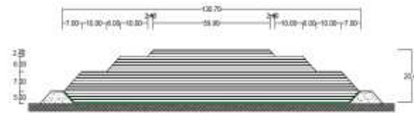
Gambar 7. Perencanaan geometri landfill .
