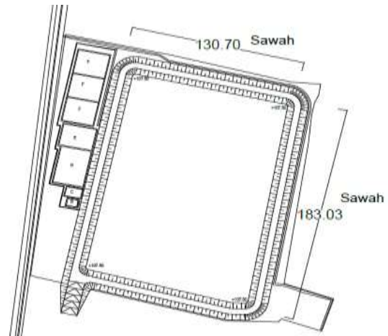
Gambar 2. Tampak atas TPA Sekoto Baru.
