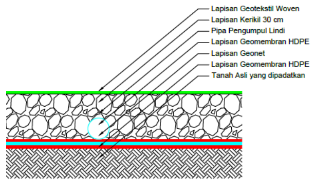
Gambar 6. Perencanaan lapisan liner TPA.
