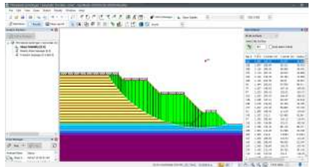
Gambar 10. Hasil analisa stabilitas overall timbunan sampah menghadap sawah.
