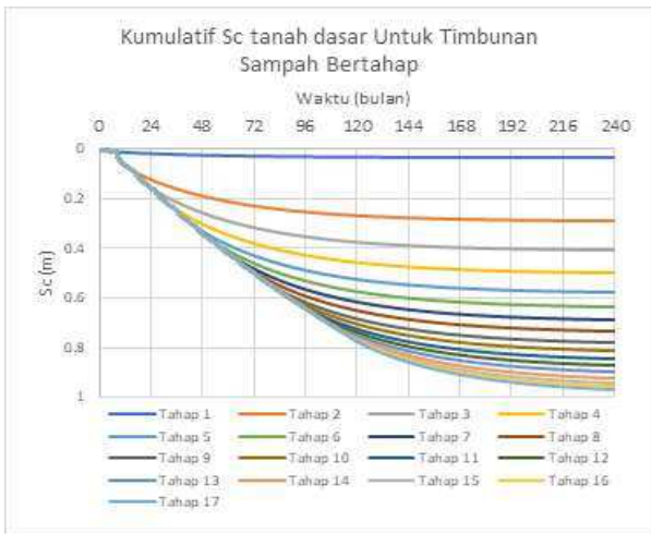
Gambar 8. Grafik hubungan besarnya settlement akibat beban bertahap sampah dengan waktu.
