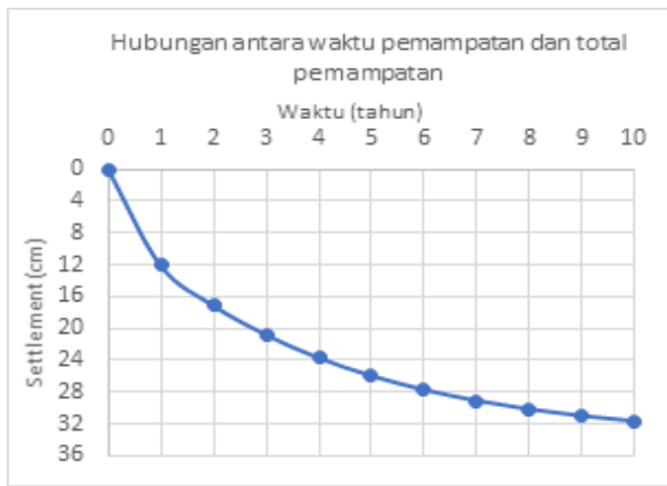
Gambar 3. Hubungan antara waktu dan total settlement akibat beban tanggul.
