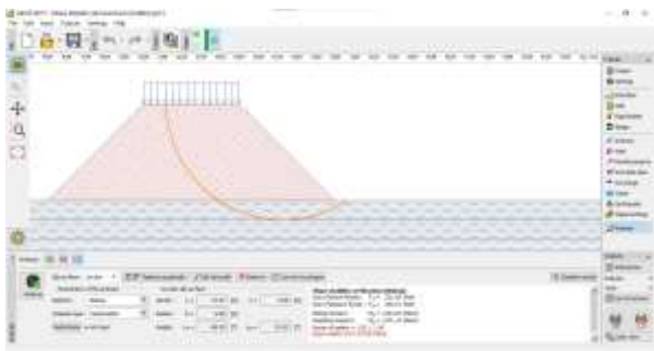
Gambar 4. Hasil analisa stabilitas tanggul.
