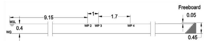
Gambar 3.11 Dimensi flume untuk validasi
