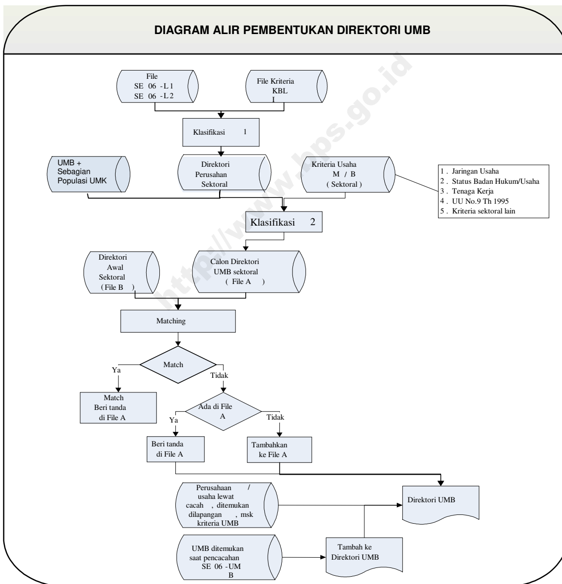
Gambar 1. Diagram Alir Pembentukan Direktori UMB
