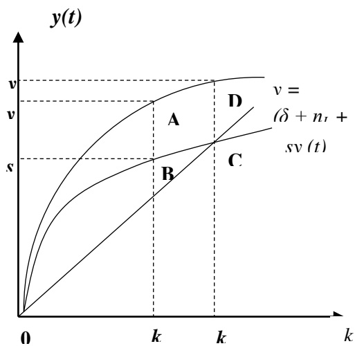
Gambar 1. Output dan Investasi pada Steady State
