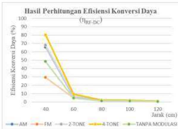
Gambar 8. Hasil perbandingan Efisiensi Konversi Daya.
