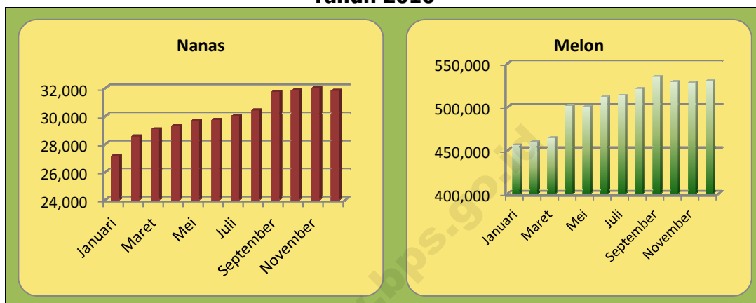
Grafik 3. Harga Produsen Nanas dan Melon Tahun 2010
