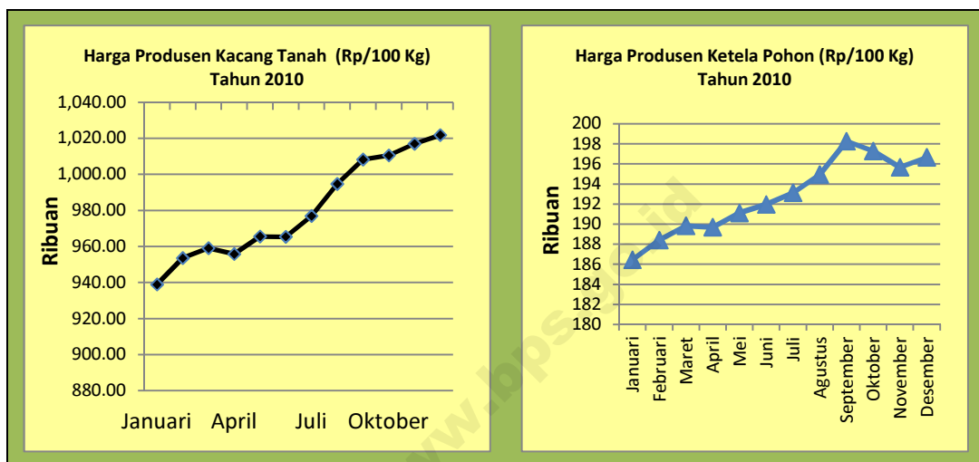
Grafik 1. Harga Produsen Kacang Tanah dan Ketela Pohon Tahun 2010
