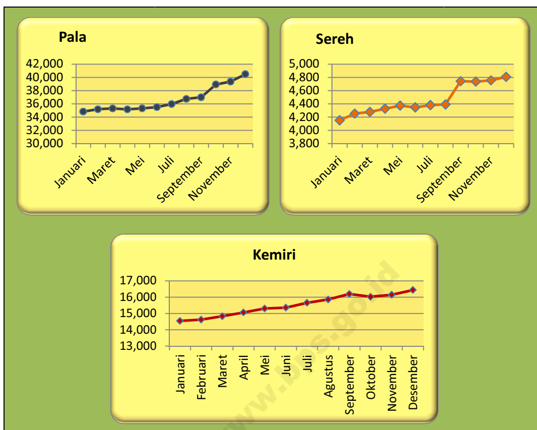
Grafik 4. Harga Produsen Pala, Sereh dan Kemiri (Rp/Kg) Tahun 2010
