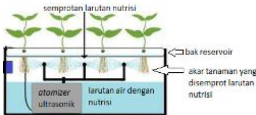
Gambar 10. Rancangan ruang tumbuh GrowBox .
