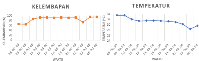
Gambar 16. Grafik pengujian DHT22.
