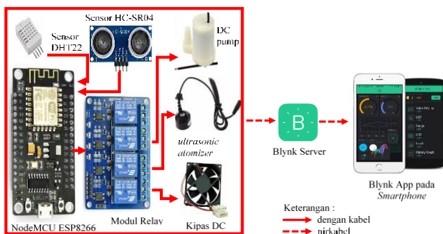
Gambar 11. Hubungan antar komponen.
