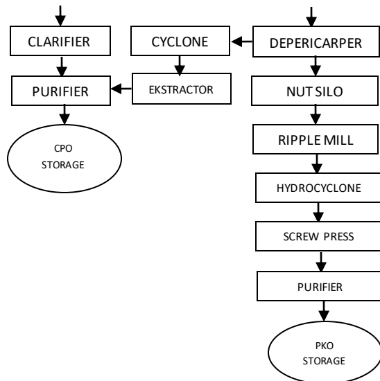
Gambar 1. Blok Diagram Skema Proses Pembuatan CPO dan PK
