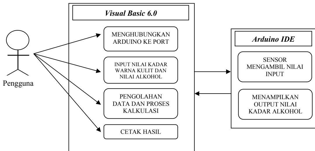
Gambar 3.1 Arsitektur Perangkat Lunak Alat Ukur Kadar Alkohol
