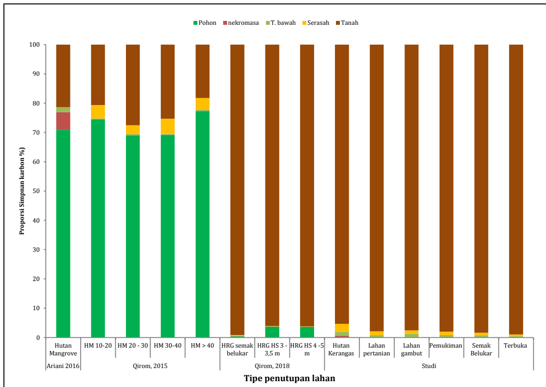
Gambar 4. Proporsi simpanan karbon pada hutan mangrove (Ariani et al. , 2016); HRG: hutan rawa gambut (Qiom et al. , 2018); dan HM: hutan mineral (Qiom et al. , 2015).
