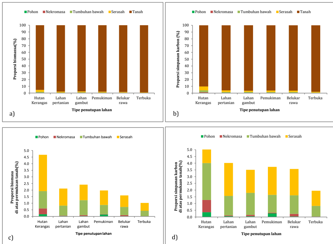
Gambar 3. Proporsi: a) biomassa total; b) simpanan karbon; c) biomassa permukaan tanah; d) karbon permukaan tanah pada masing-masing komponen karbon di penutupan lahan yang berbeda
