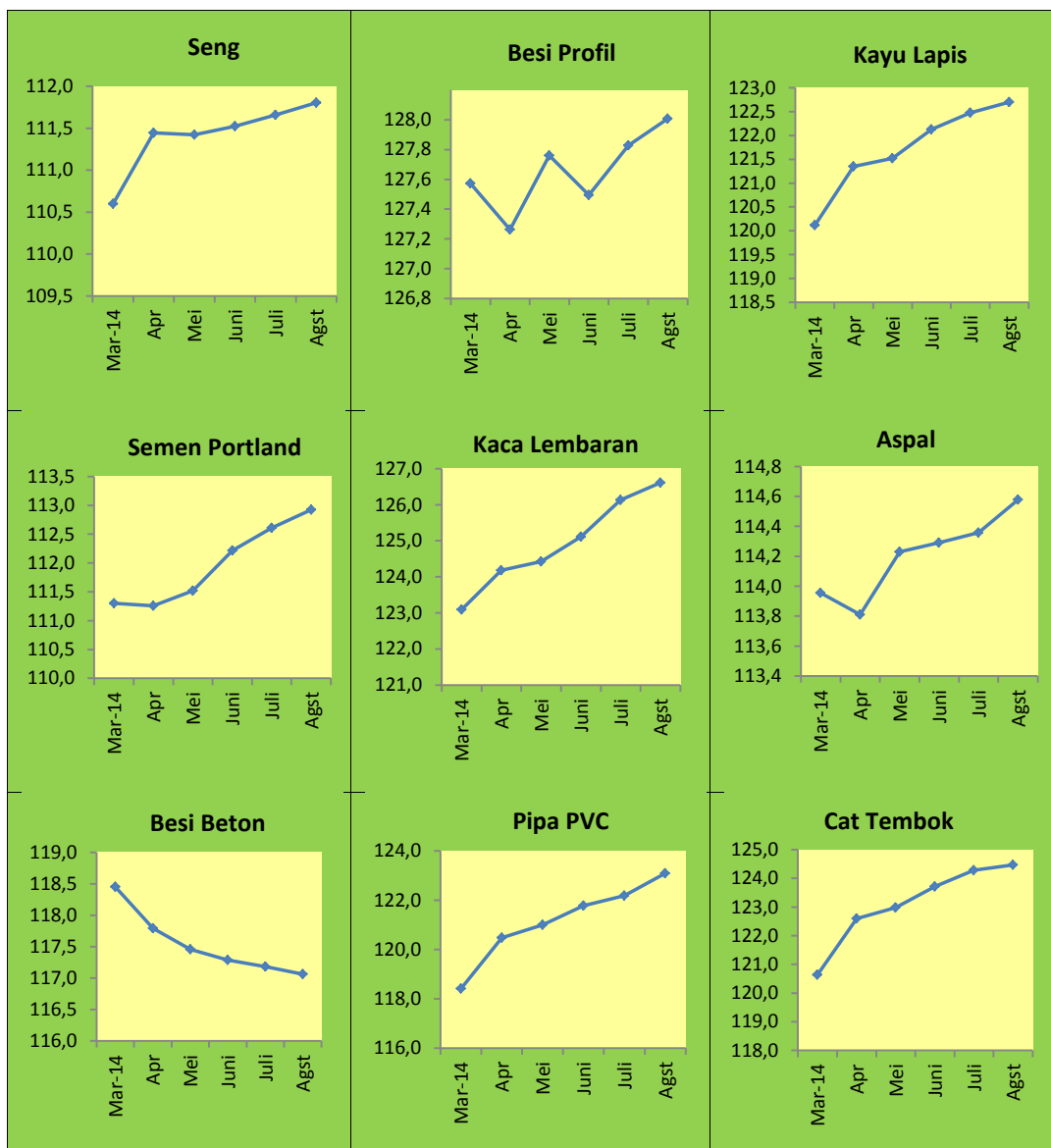
Grafik 10.3 Indeks Harga Beberapa Bahan Bangunan, Maret–Agustus 2014
