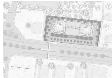
Gambar 16. Site Plan.
