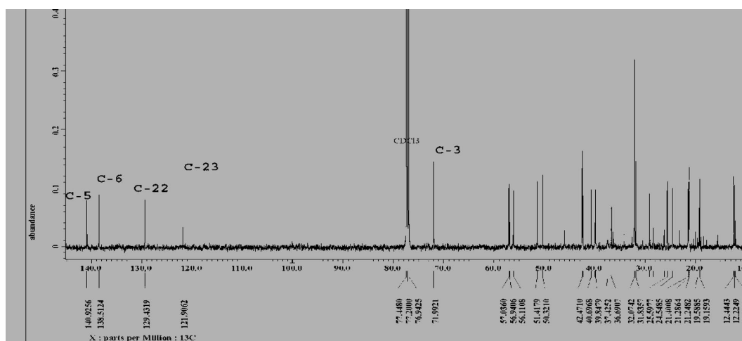
Gambar 3. Spektrum ^{13}C -NMR senyawa 1 yang diperoleh dari ekstraksi akar Garcinia cowa Roxb. ex pada 125 MHz ( CDCl_3 )
