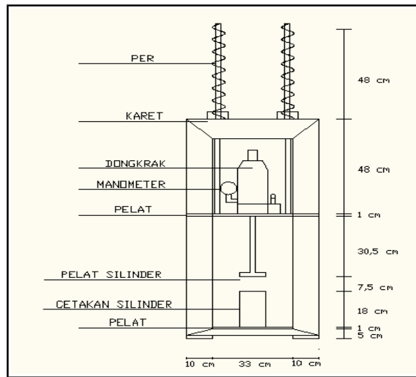
Gambar 2. Sketsa alat uji tekan modifikasi.
