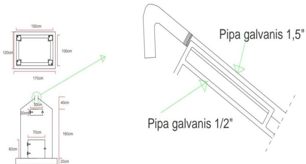
Gambar 1. Design Bangunan Instalasi Pengolah Cuka Kayu
