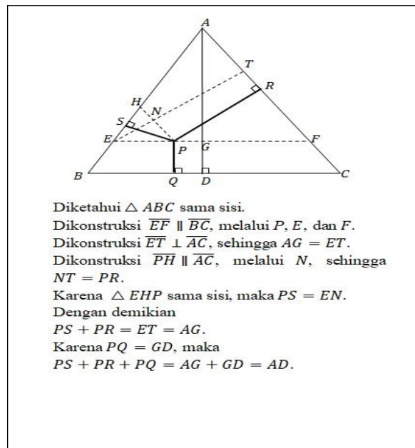
Gambar 2. Pembuktian Teorema Viviani Cara II
