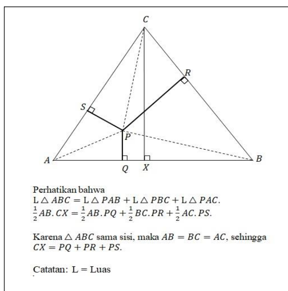
Gambar 1. Pembuktian Teorema Viviani Cara I
