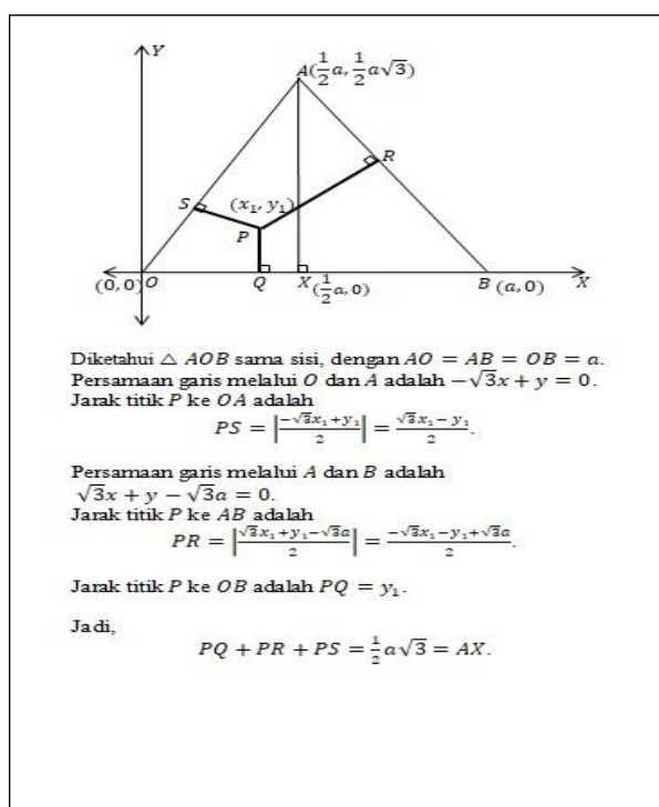
Gambar 3. Pembuktian Teorema Viviani Cara III
