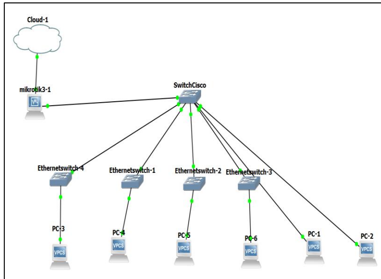
Gambar 7. Hasil implementasi jaringan
