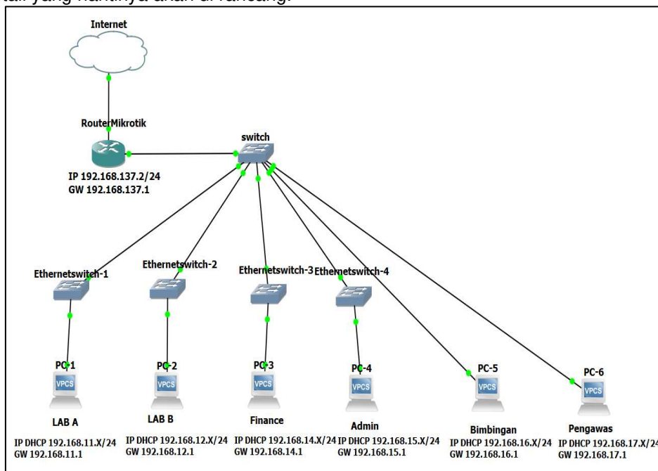
Sumber: Rumah Shalom Mahanaim (2019) Gambar 4. Arsitektur jaringan berjalan
