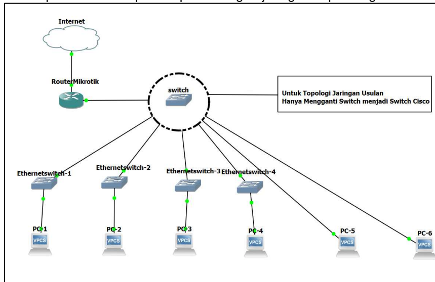
Gambar 5. Topologi Jaringan Usulan
