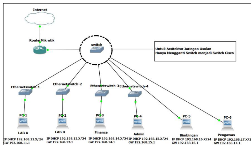
Gambar 6. Arsitektur jaringan usulan
