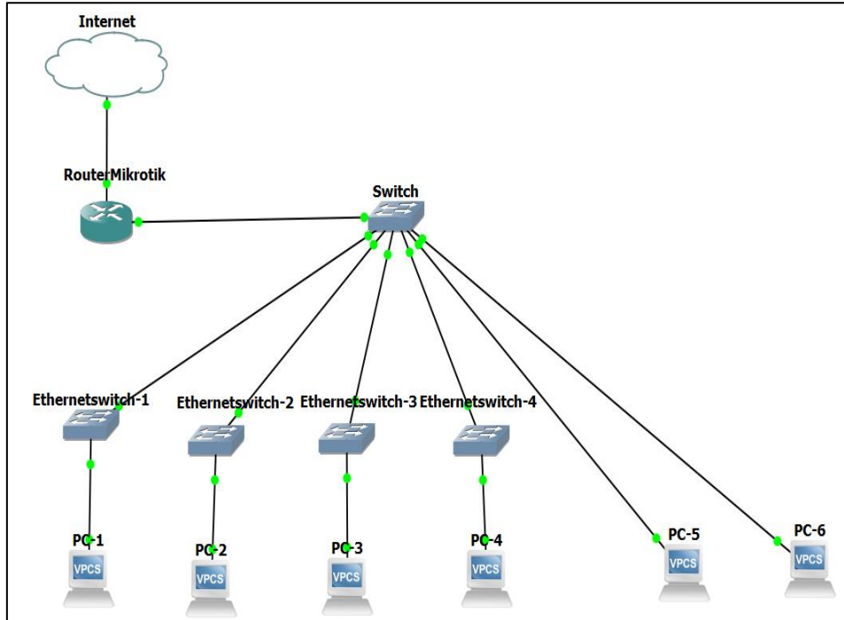
Sumber: Rumah Shalom Mahanaim (2019) Gambar 3. Topologi jaringan berjalan
