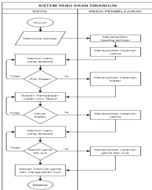
Gambar 3. Flowmap Sistem Yang Akan Dibangun
