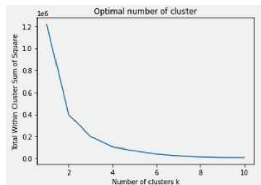
Gambar 4. Penentuan jumlah cluster menggunakan metode Elbow
