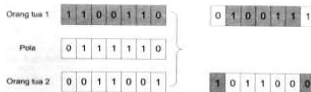
Gbr. 4 Pindah silang pola seragam.
