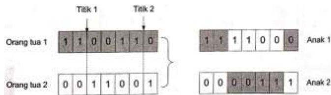
Gbr. 3 Pindah silang banyak titik.
