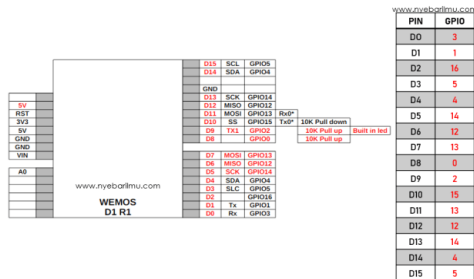
Gambar 2.5 Penentuan GPIO dari board Wemos D1 R1
