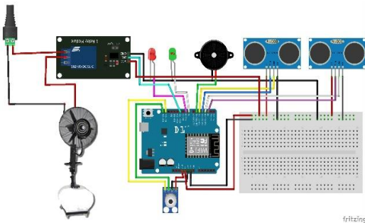
Gb. 2.2 Perancangan Perangkat keras
