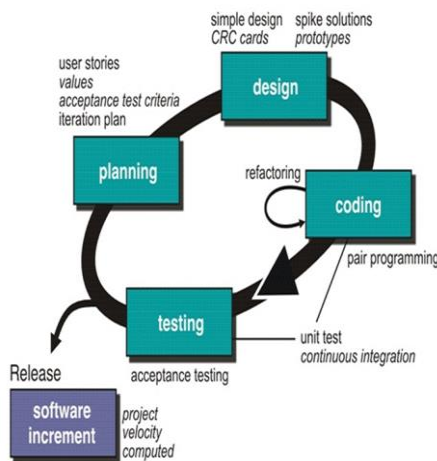
Gambar 1. Kerangka Kerja XP Sumber : Syafitri, Y. (2016), jurnal cendikia [6]
