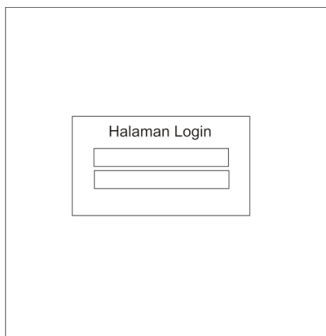
Gambar 4 . Tampilan Login
