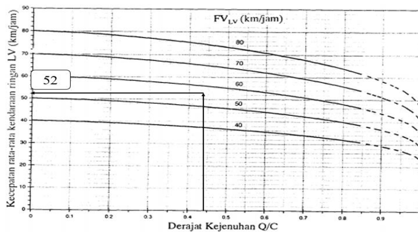
Gambar 1. Nilai kecepatan untuk fungsi dari DS pada ruas jalan banyak-lajur dan satu arah
