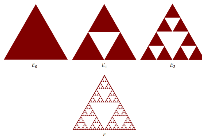
Gambar 4. Konstruksi segitiga Sierpinski.
