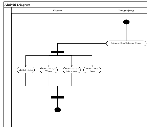
Gambar 9. Activity Diagram Pengunjung
