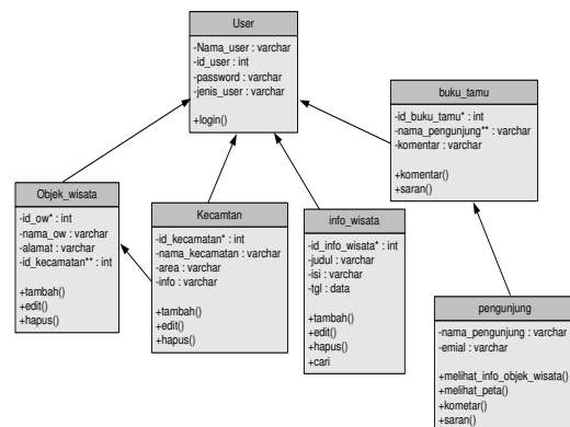
Gambar 3. Class Diagram SIG
