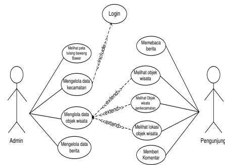
Gambar 2. Usecase Sistem
