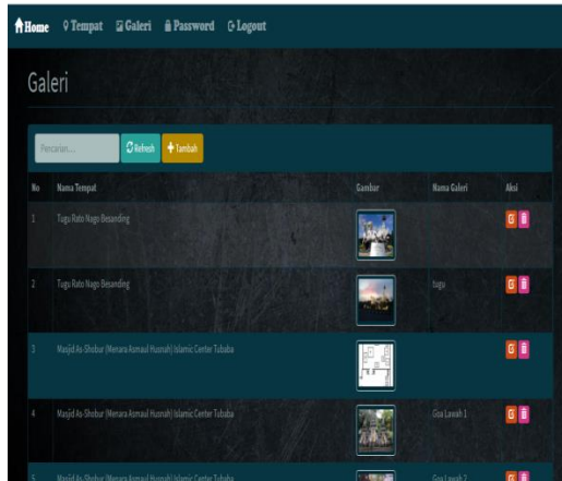
Gambar13. HalamanGaleriAdmin
