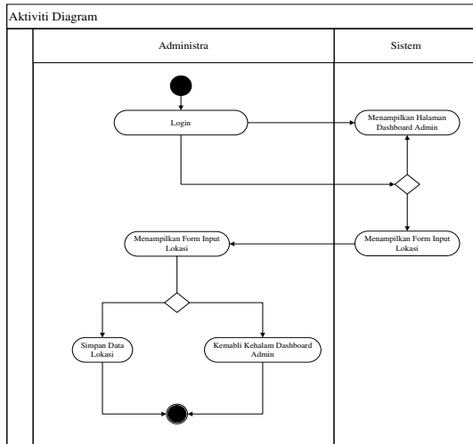
Gambar 8. Activity Diagram Tempat Wisata+
