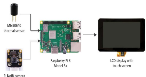
Gambar 3 Blok Diagram Sistem Elektronik
