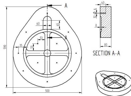
Gambar 6. Dimensi cetakan bawah dalam satuan
