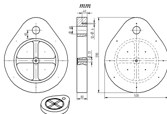
Gambar 7. Dimensi cetakan atas dalam satuan mm
