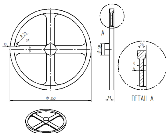
Gambar 5. Dimensi pola pulley dalam satuan mm
