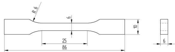
Gambar 10. Dimensi spesimen uji tarik
