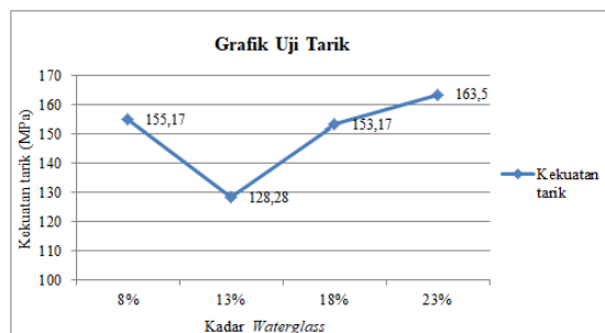
Gambar 12. Grafik pengaruh kadar waterglass terhadap nilai kekuatan tarik
