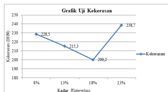
Gambar 11. Grafik pengaruh kadar waterglass terhadap nilai kekerasan
