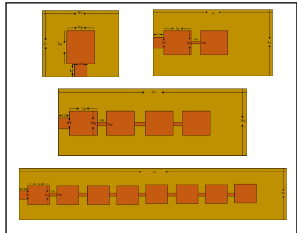
Gambar 4. Desain antenna 1x1, 1x2, 1x4 dan 1x8.
