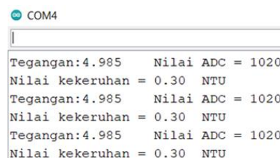
Gambar 12. Hasil Kalibrasi Sensor Kekeruhan
