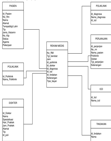
Gambar 8. Tabel relasi
