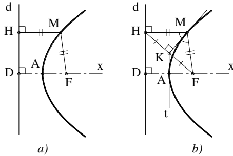
Hình 1. Parabola và các đặc điểm
