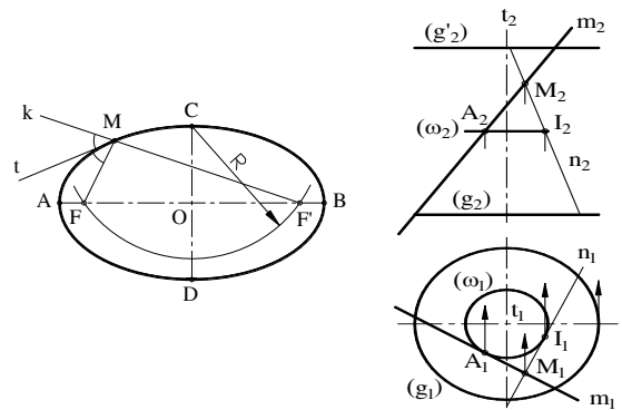
Hình 4. Vẽ tiếp tuyến với elip tại điểm thuộc elip
