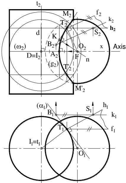
Hình 6. Giao tuyến của mặt cầu và mặt trụ tròn xoay
