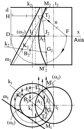
Hình 13. Giao tuyến của mặt trụ và hyperboloid tròn xoay
