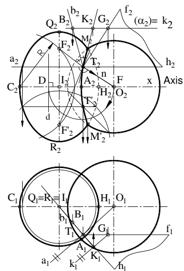
Hình 12. Giao tuyến của mặt elipxoid tròn xoay và cầu
