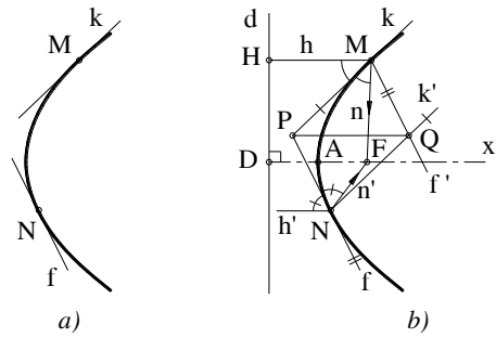
Hình 3. Xác định phương của trục parabola
