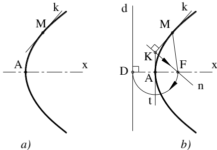
Hình 2. Xác định các đặc trưng của parabola
