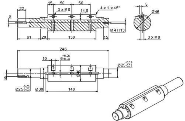
Hình 15. Thiết kế 2D trục gá dao cắt
