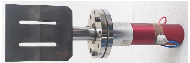
Hình 18. Hệ siêu âm 20 kHz thực tế
