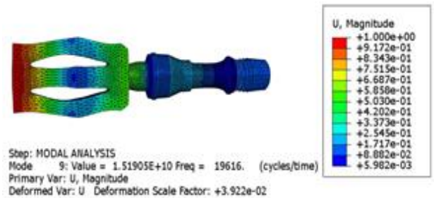
Hình 16. Biên độ dao động siêu âm 20 kHz
