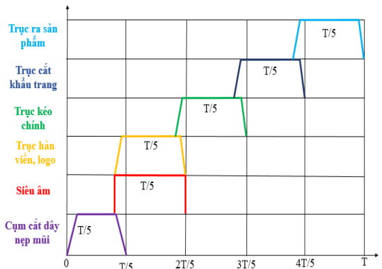
Hình 6. Biểu đồ trạng thái hoạt động 1 chu kỳ T
