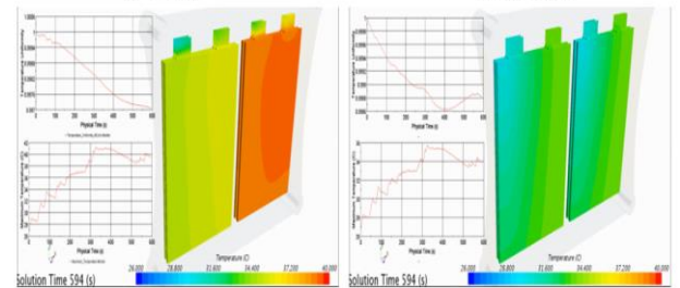
Hình 23b. Mô phỏng so sánh hiệu quả làm mát bằng khí và bằng nước cho pin Li-Ion
