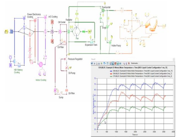
Hình 28. Hệ thống làm mát bằng dung dịch cho xe điện và hiệu quả làm mát động cơ của 3 cấu hình thiết kế khác nhau
