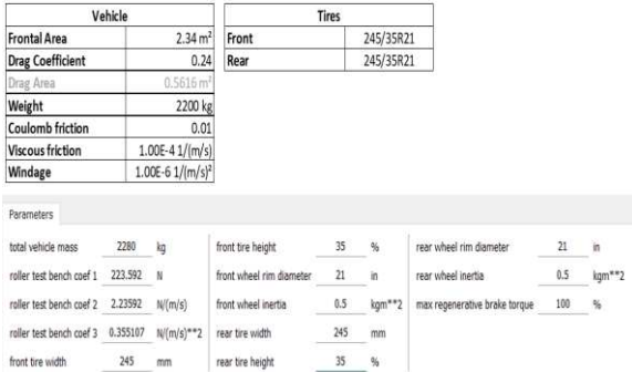
Hình 9. Các thông số mô hình của xe Tesla model SP85 xây dựng trên Amesim
