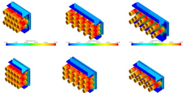
Hình 23a. Thuật toán tối ưu trong mô phỏng nhiệt khối pin Li-Ion Air Cooling Water Cooling
