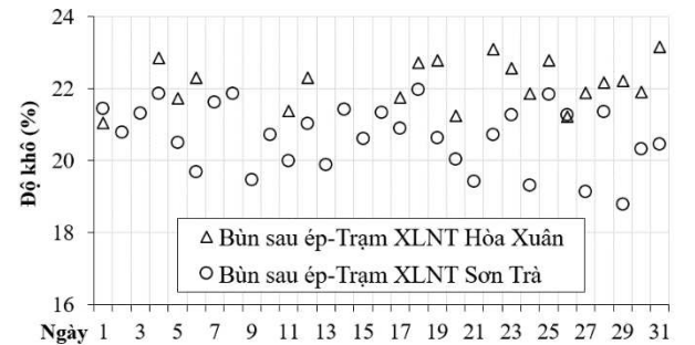
Hình 7. Độ khô của bùn sau ép tại trạm Hòa Xuân và Sơn Trà
