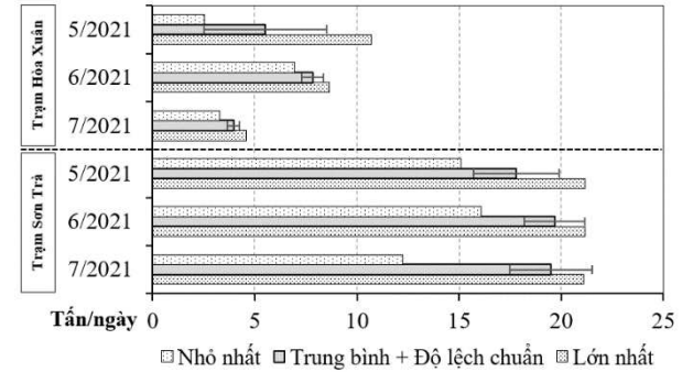
Hình 6. Lượng bùn xử lý thống kê trong 3 tháng tại hai trạm
