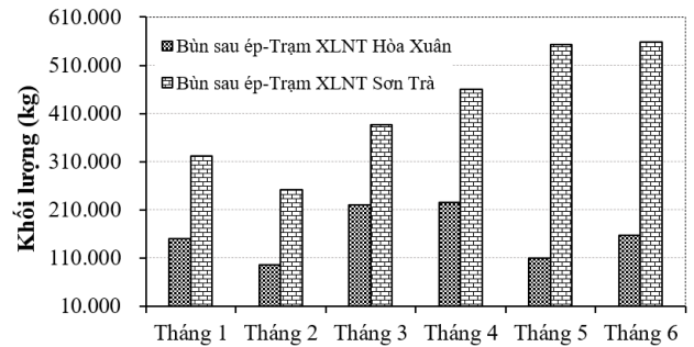
Hình 8. Lượng bùn xử lý tại KXL Khánh Sơn
