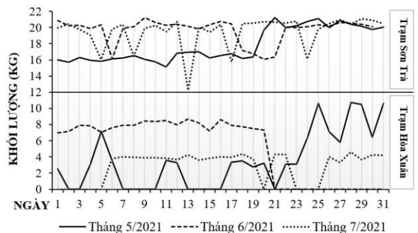
Hình 5. Lượng bùn sau ép trong 3 tháng tại hai trạm
