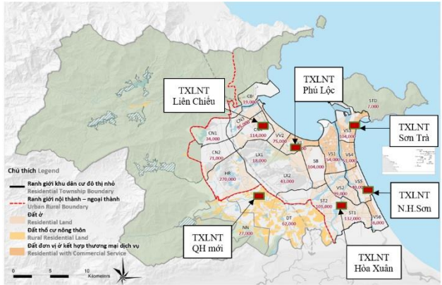
Hình 1. Bản đồ vị trí các trạm XLNT đô thị tại Đà Nẵng Trạm XLNT Sơn Trà là nhà máy được đầu tư chuyển đổi công nghệ XLNT hồ yếm khí có phủ bạt kín do Ngân hàng thế giới tài trợ từ năm 2008 và trạm XLNT Hòa Xuân được quy hoạch xây dựng mới, là 02 đối tượng lựa chọn nghiên cứu điển hình tại thành phố Đà Nẵng. Nguồn nước thải, công suất xử lý và sự khác biệt về công nghệ XLNT là các tiêu chí quan tâm khi lựa chọn đối tượng khảo sát, đánh giá. Thông tin cơ bản về 02 trạm XLNT được trình bày tại Bảng 1.
