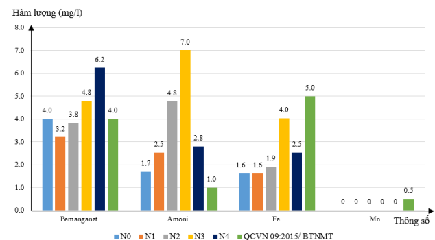
Hình 4. Biểu đồ phân tích kết quả mẫu nước dưới đất tại khu vực bãi rác Cẩm Hà
