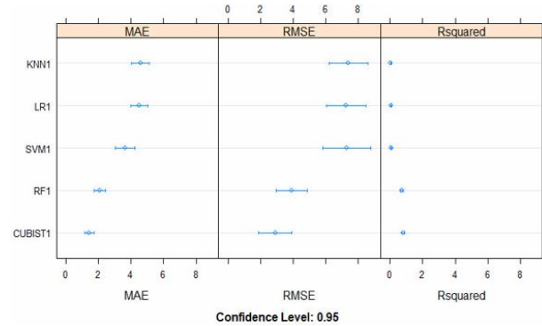
Hình 5. Biểu đồ kết quả từ dữ liệu Training với tỷ lệ 70:30
