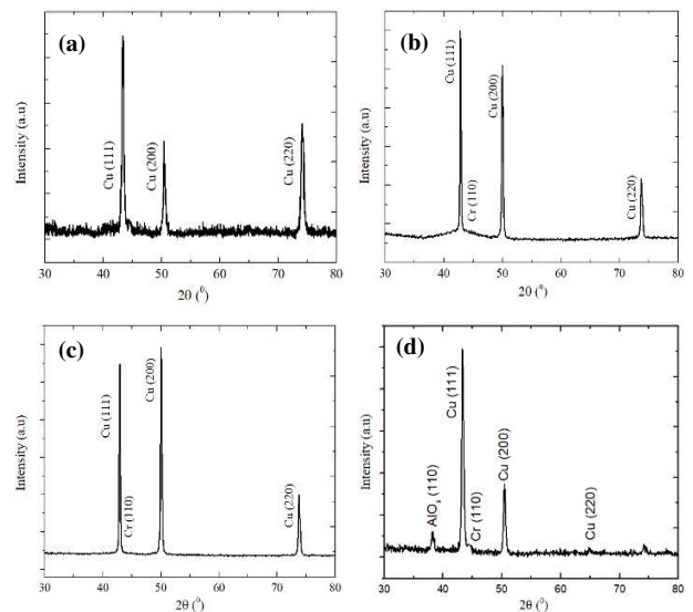
Hình 8. Phân tích XRD cho (a) vật liệu nền và lớp mạ thu được từ dung dịch mạ (b) S_{Na4} ; (c) S_{Mg4} và (d) S_{Al4} . Điều kiện: pH = 1,7; hiện hành mật độ A/dm 2 , T = 30°C, thời gian = 15 phút
