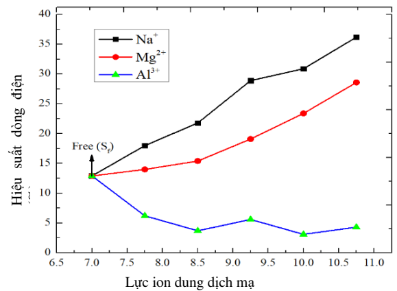
Hình 7. Ảnh hưởng của lực ion đến hiệu suất dòng điện trong quá trình mạ điện Crom sử dụng dung dịch mạ Cr(III) có lực ion từ 7,75 đến 10,75. Điều kiện: pH = 1,7; hiện hành mật độ 5A/dm 2 , T = 30°C, thời gian = 15 phút
