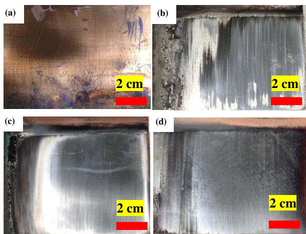
Hình 3. Hình ảnh chụp bằng hiển vi quang học cho lớp mạ Crom thu được từ dung dịch mạ khác nhau:
