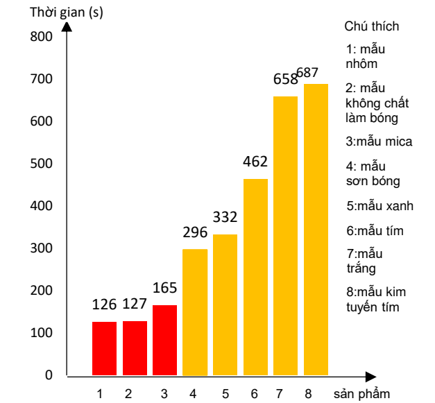
Hình 4. Đồ thị hiển thị tốc độ bay hơi của dung môi
