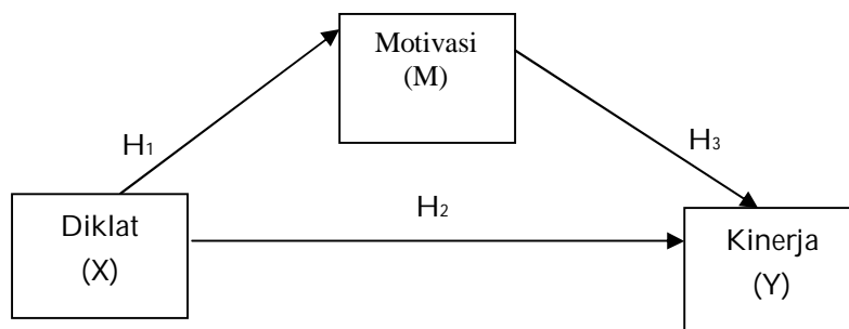
Gambar 1 Kerangka Konsep Penelitian
