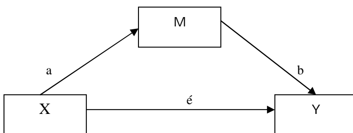
Gambar 2 Struktur 1 Hubungan Langsung X Mempengaruhi Y Struktur 2 Hubungan Tidak Langsung X Mempengaruhi Y, Melalui M
