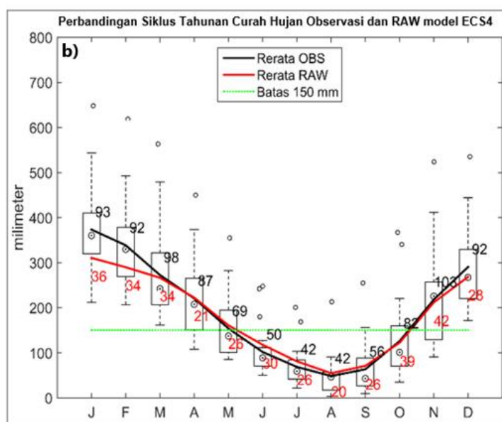
Gambar 1. (a) Lima kategori reliabilitas berdasarkan bentuk kurva Reliability Diagram (dimodifikasi dari Weisheimer and Palmer, 2014 dan (b) Rerata siklus tahunan curah hujan dari semua stasiun BMKG di P. Jawa untuk observasi (hitam), RAW model ECS4 (merah) dengan angka pada garis adalah standar deviasi tiap bulan. sedangkan rerata curah hujan bulanan untuk observasi tiap stasiun ditampilkan dalam bentuk boxplot. Batas pembeda musim kemarau dan musim hujan ditunjukkan oleh garis horizontal hijau putus-putus pada nilai 150 mm/bulan.
