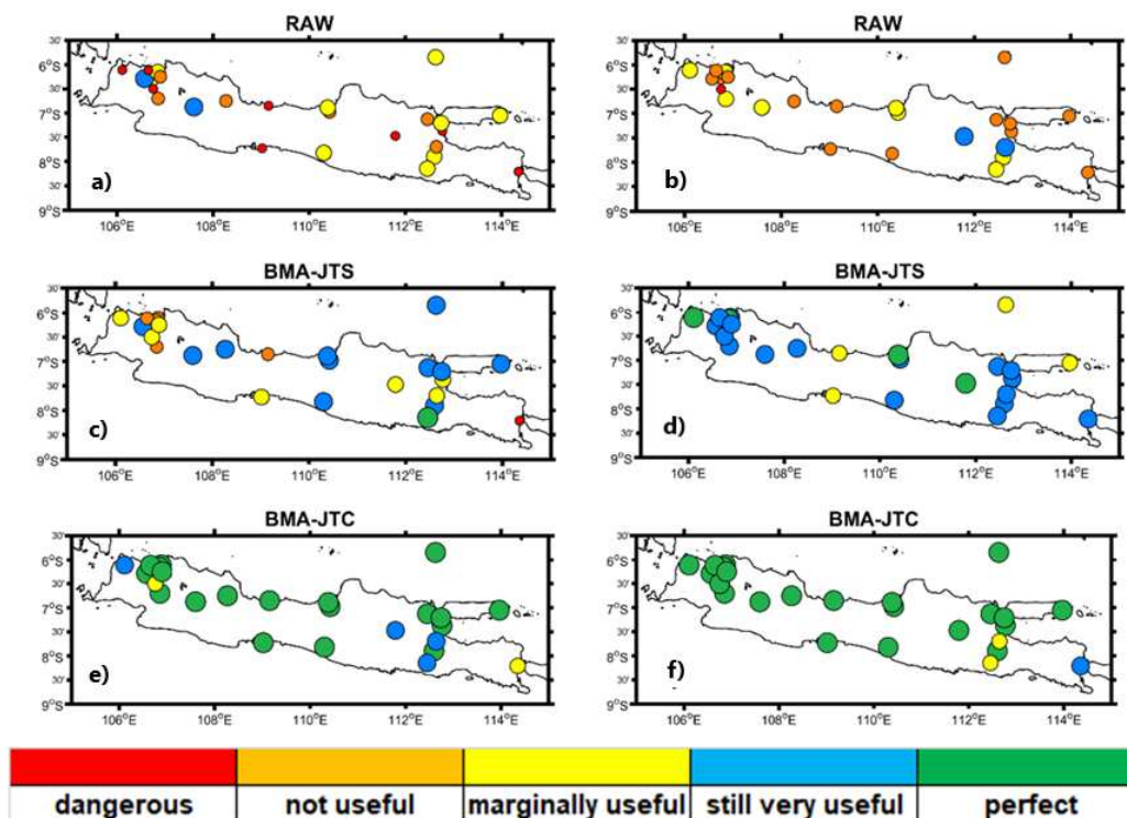
Gambar 6. Perbandingan kategori Reliability Diagram : RAW model ECS4 (a, b), hasil kalibrasi BMA-JTS (c, d) dan BMA-JTC (e, f) untuk prediksi probabilistik kejadian BN (kolom kiri) dan AN (kolom kanan)
