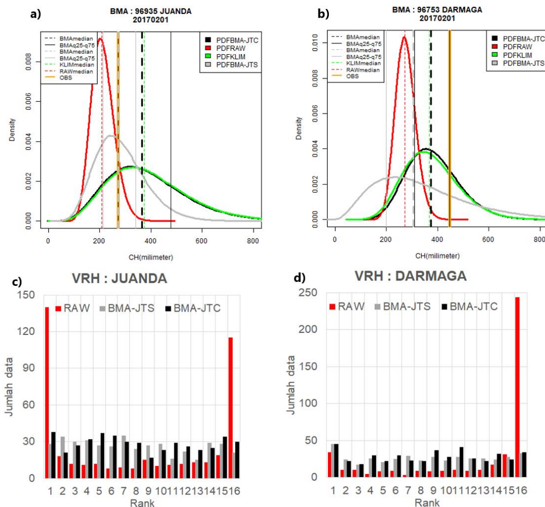
Gambar 3. Panel a dan b: PDF BMA-JTS (abu-abu), BMA-JTC (hitam), PDF RAW model (merah), PDF klimatologi (hijau), observasi (garis vertikal orange) untuk Februari 2017; Panel c dan d: VRH BMA-JTS ( bar abu-abu), VRH BMA-JTC (hitam) dan VRH RAW model (merah). Kolom kiri (kanan) untuk stasiun Juanda (Darmaga).
