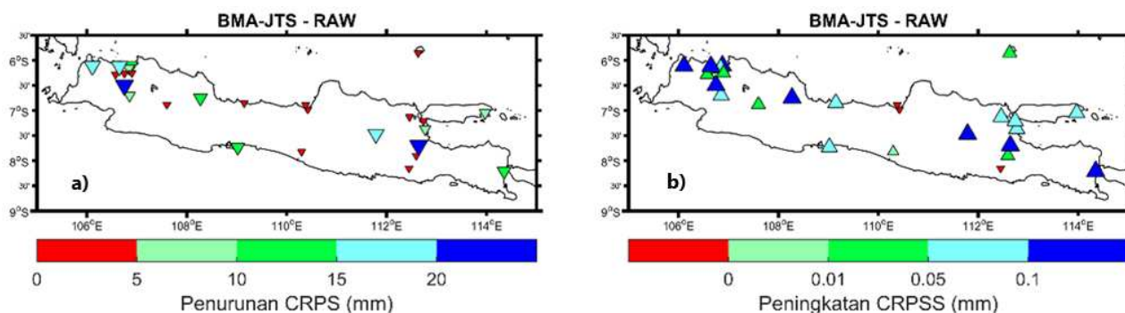
Gambar 4. Penurunan nilai Continous Rank Probability Source (CRPS) (a) dan peningkatan skill CRPS (b) hasil BMA-JTS dengan JT 30 bulan terhadap RAW model ECS
