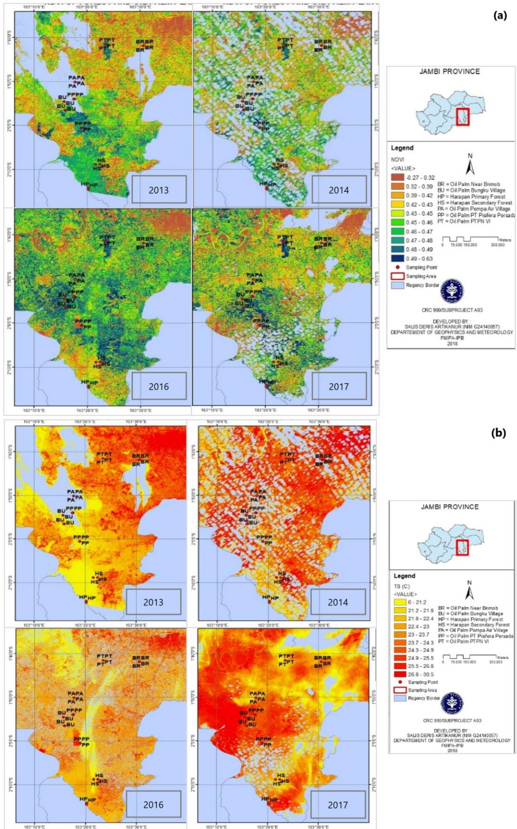
Gambar 1. Hasil pengolahan data citra Landsat 8 untuk parameter (a) NDVI, dan (b) suhu permukaan pada tutupan lahan hutan dan perkebunan kelapa sawit di Jambi tahun 2013, 2014, 2016, dan 2017. BR titik sampel untuk KS2 (kelapa sawit umur 2 tahun), PP1 titik sampel untuk KS3 (kelapa sawit umur 3 tahun), PA titik sampel untuk KS7 (kelapa sawit umur 7 tahun), BU1 titik sampel untuk KS7.5 (kelapa sawit umur 7.5 tahun), BU2 titik sampel untuk KS15 (kelapa sawit umur 15 tahun), PT titik sampel untuk KS19 (kelapa sawit umur 19 tahun), PP2 titik sampel untuk KS28 (kelapa sawit umur 28 tahun), HS titik sampel untuk hutan sekunder, HP titik sampel untuk hutan primer.
