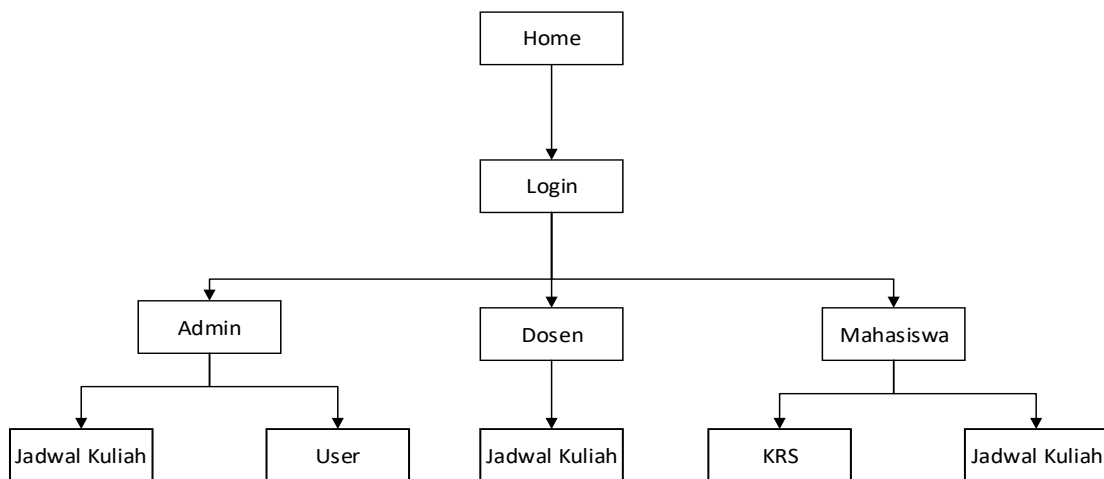
Gambar 4. Struktur Menu
